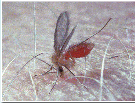
รูปร่างของรึ้นฝอยทราย
