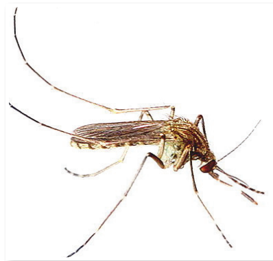
ยุงรำคาญชนิด Culex tritaeniorhynchus ซึ่งเป็นพาหะนำโรคไข้สมองอักเสบ
